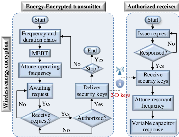
Fig. 5. 2-D chaotic FDE scheme.
