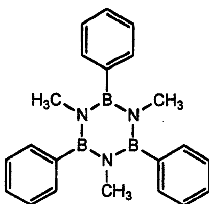
化合物 4
