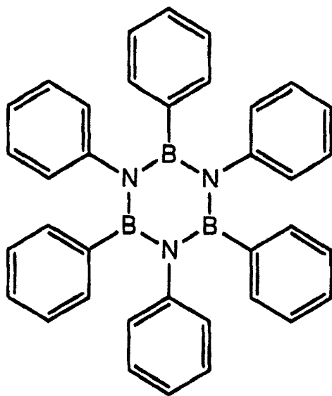
化合物 6
