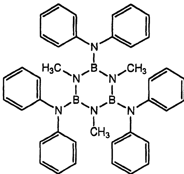
化合物 7
