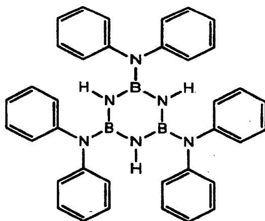
化合物 3
