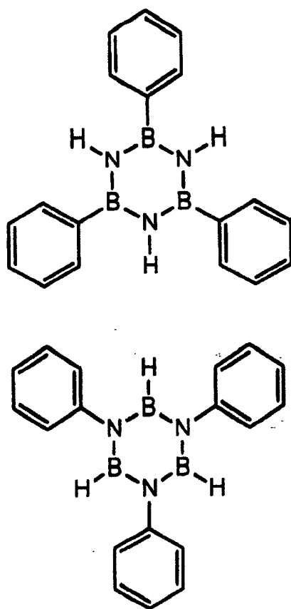
化合物 2
