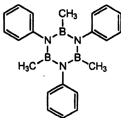
化合物 4
