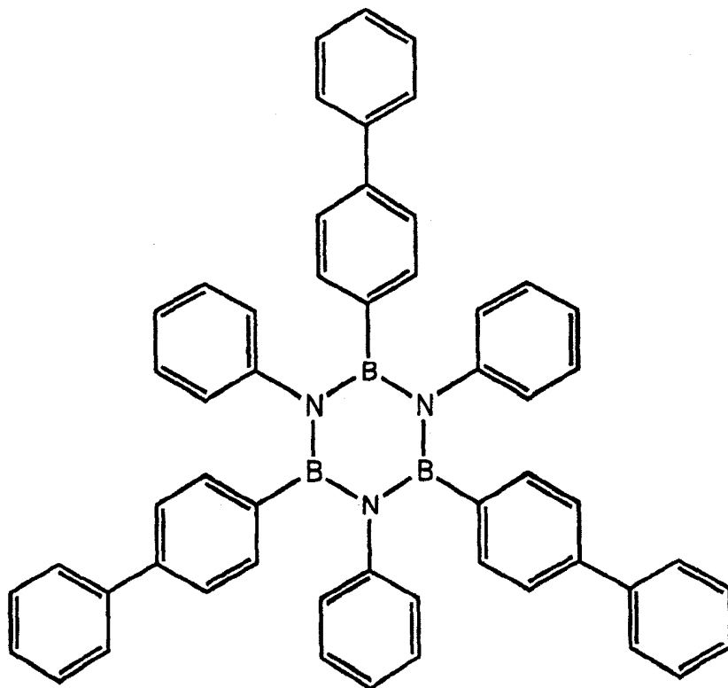
化合物 10
