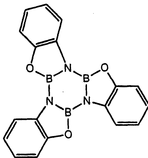
化合物 11
