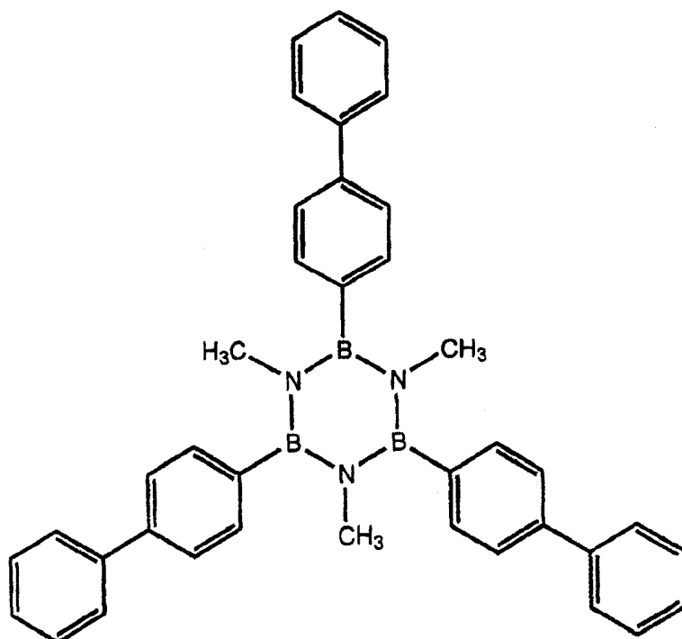
化合物 9
