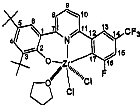
催化剂 6
