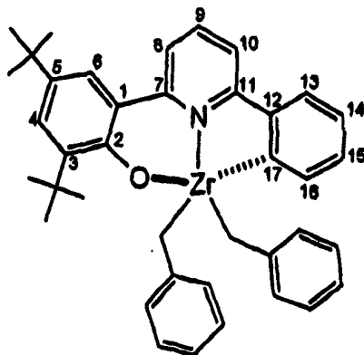
催化剂 1
