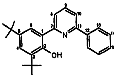
中间体 2
