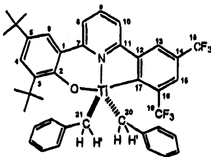
催化剂 4
