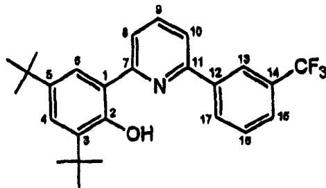
中间体 4
