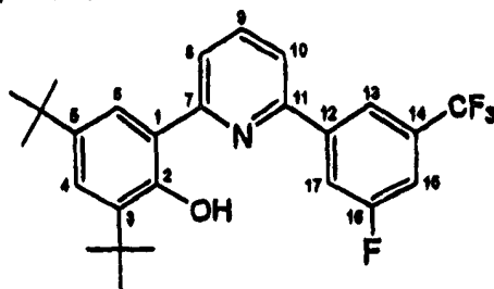
中间体 5
