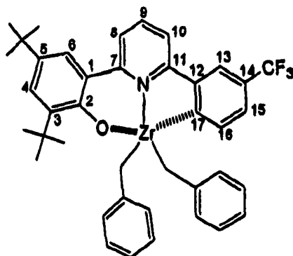
催化剂 5
